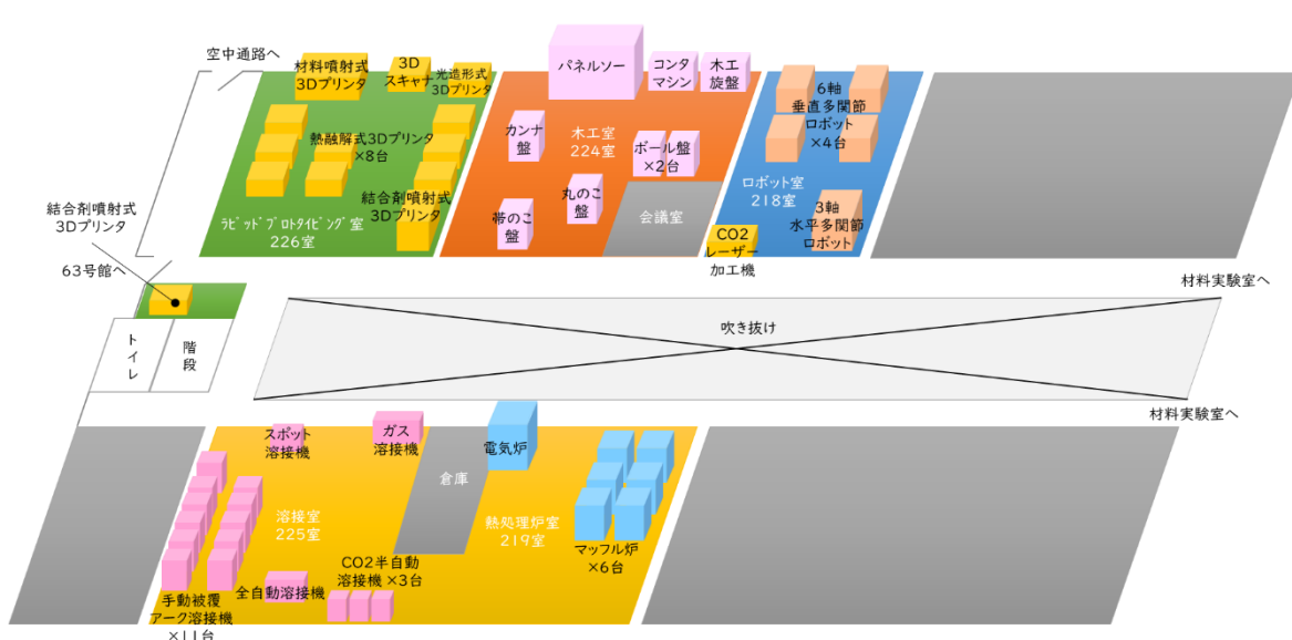
工作実験室（59号館2F西側）機械配置図
